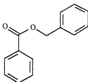
69 : Benzoato de benzila
