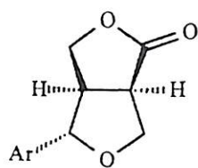
57 : Ar = Me - Glaberina
