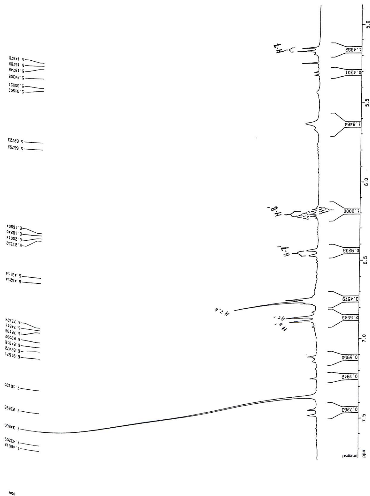
Figura 31 : Espectro de RMN de ^1\text{H} , região 4,8-7,8 ppm da neolignana V (500 MHz, \text{CDCl}_3 )
