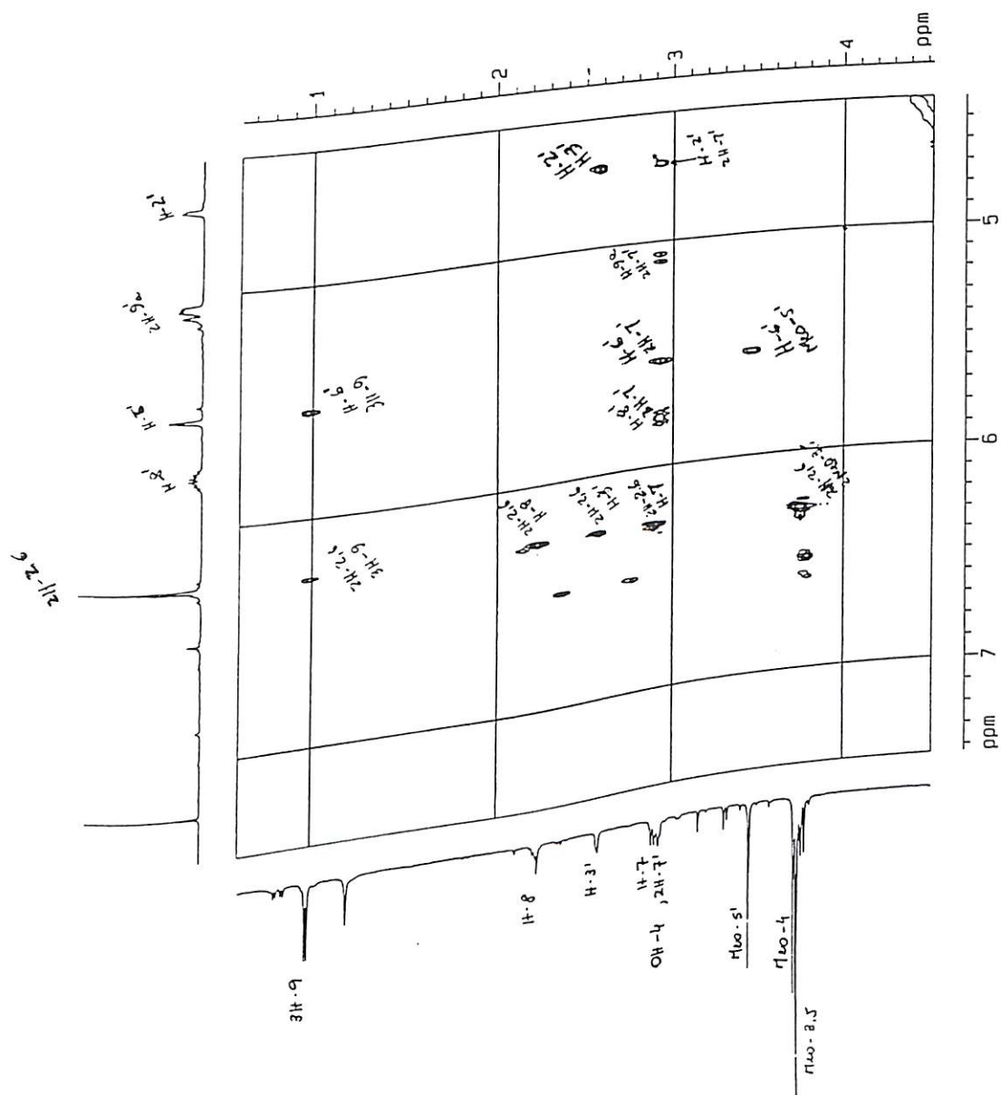
Figura 72 : Espectro de NOESY, região 4,5-7,4 x 0,7-4,5 da neolignana VII (500 MHz, CDCl 3 )
