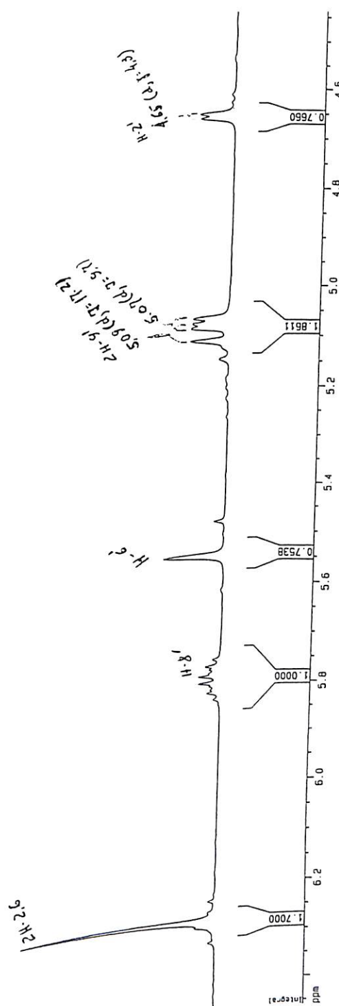
Figura 61 : Espectro de RMN ^1\text{H} , região 4,5-6,45 ppm da neolignana VII (500 MHz, \text{CDCl}_3 )
