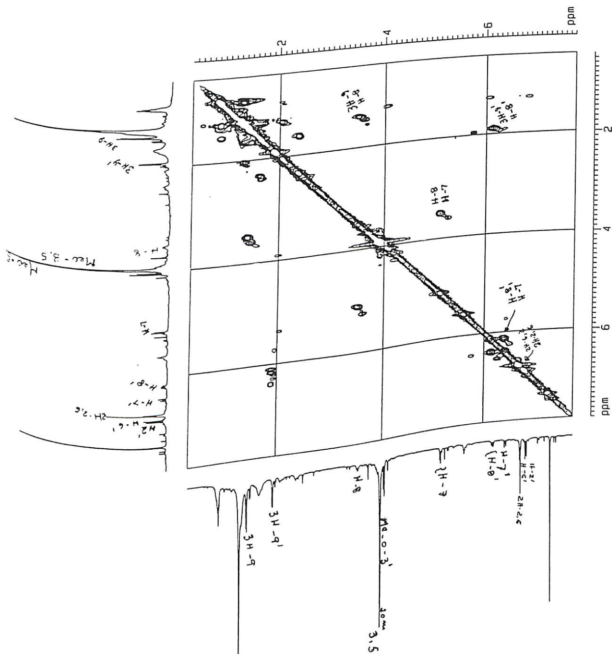
Figura 35: Espectro de RMN 2D HOMOCOSY, região 0,0-8,0 x 0,0-8,0 ppm da neolignana V (500 MHz, CDCl 3 )
