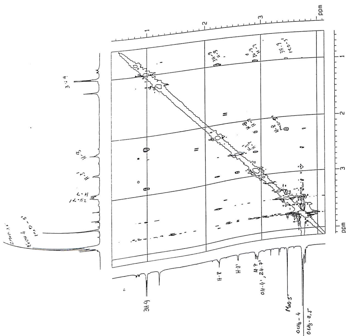
Figura 71 : Espectro de NOESY, região 1,5-4,0 x 0,5-4,0 da neolignana VII (500 MHz, \text{CDCl}_3 )
