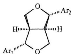
58 : Ar 1 = Ar 2 = Ve - Metilpiperitol
