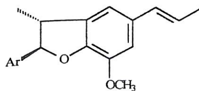
40 : Ar = Tp - Licarina C 41 : Ar = Gu - Licarina A 42 : Ar = Pi - Licarina E
