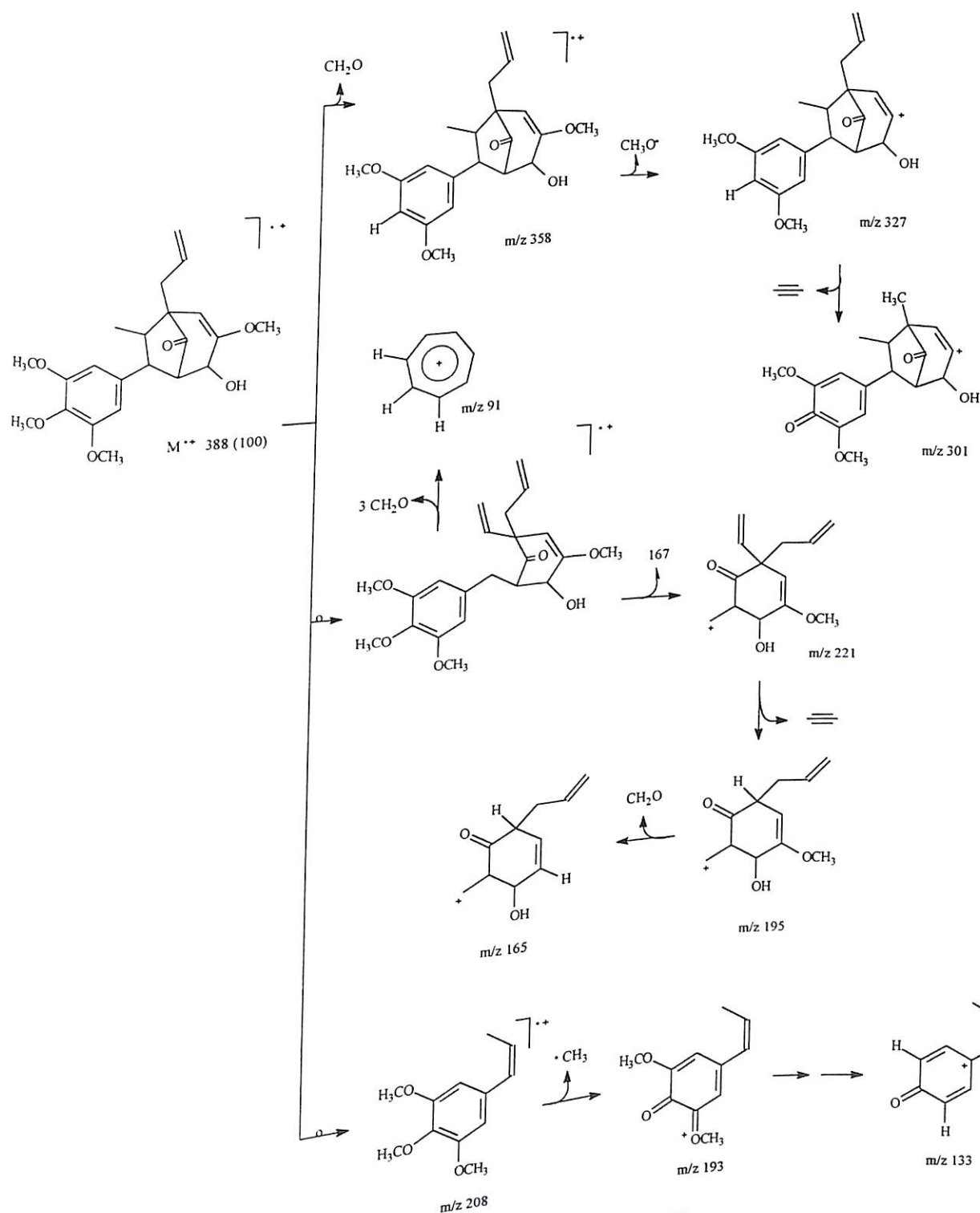
Esquema 5 : Proposta de fragmentação para a substância VIII.
