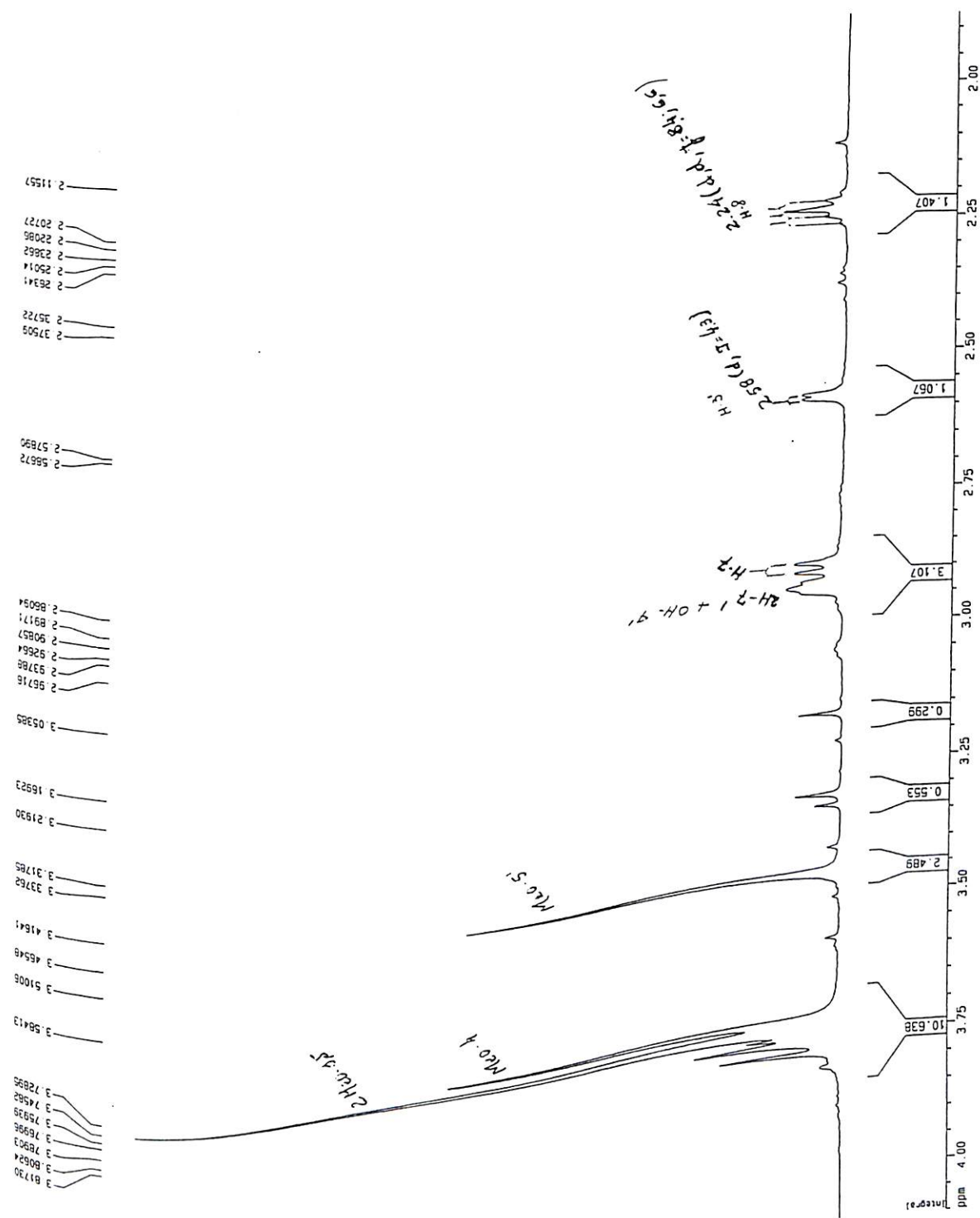
Figura 60 : Espectro de RMN ^1\text{H} , região 1,9-4,10 ppm da neolignana VII (500 MHz, \text{CDCl}_3 )
