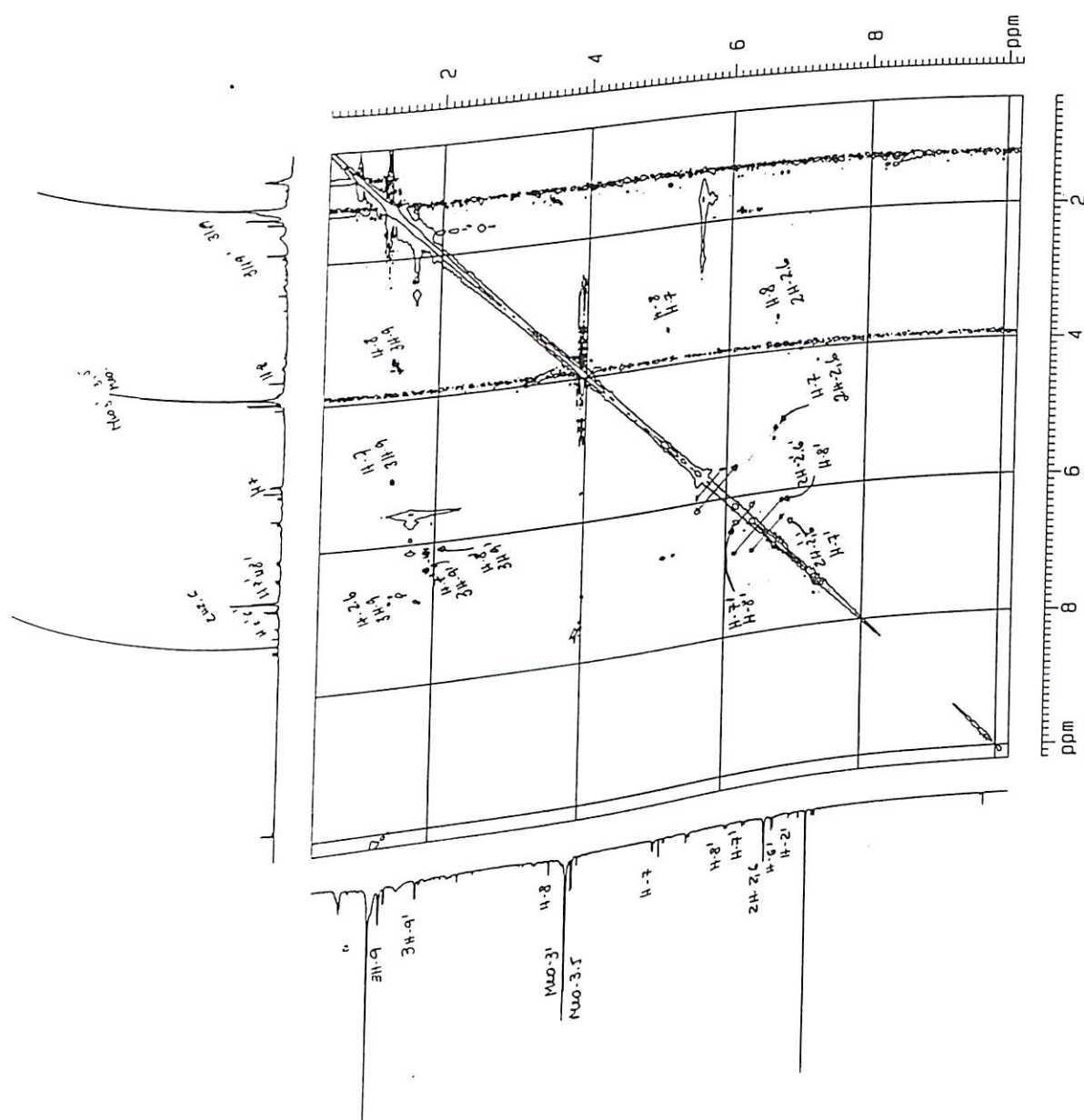
Figura 43 : Espectro de NOESY, região 0,4-10,0 x 0,4-10,0 ppm da neolignana V (500 MHz, \text{CDCl}_3 )
