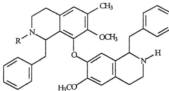
38a : 12 e 11' (-H); R = CH 3 - Ocotina 38b : 12 - 11' (-O-); R = -H - Seperina
