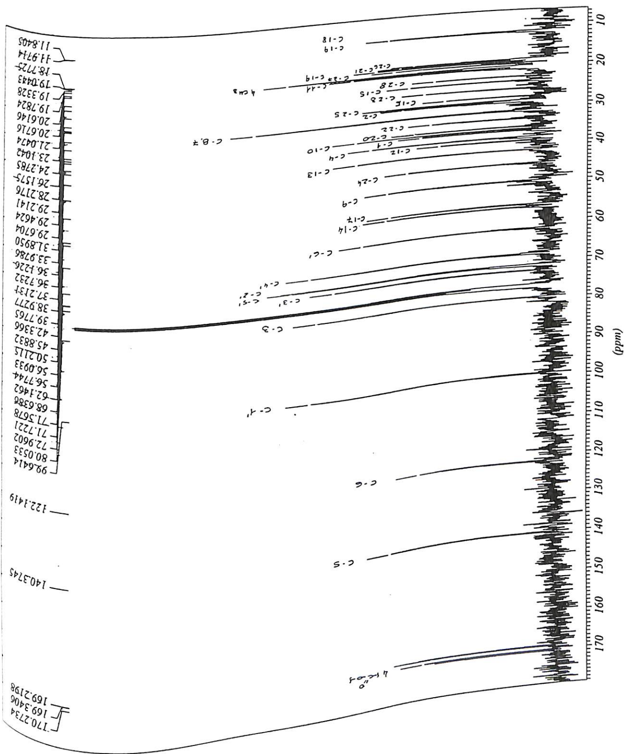
Figura 50 : Espectro de RMN de ^{13}\text{C} , região 0,7-180,0 ppm do esteróide VI (100 MHz, \text{CDCl}_3 )
