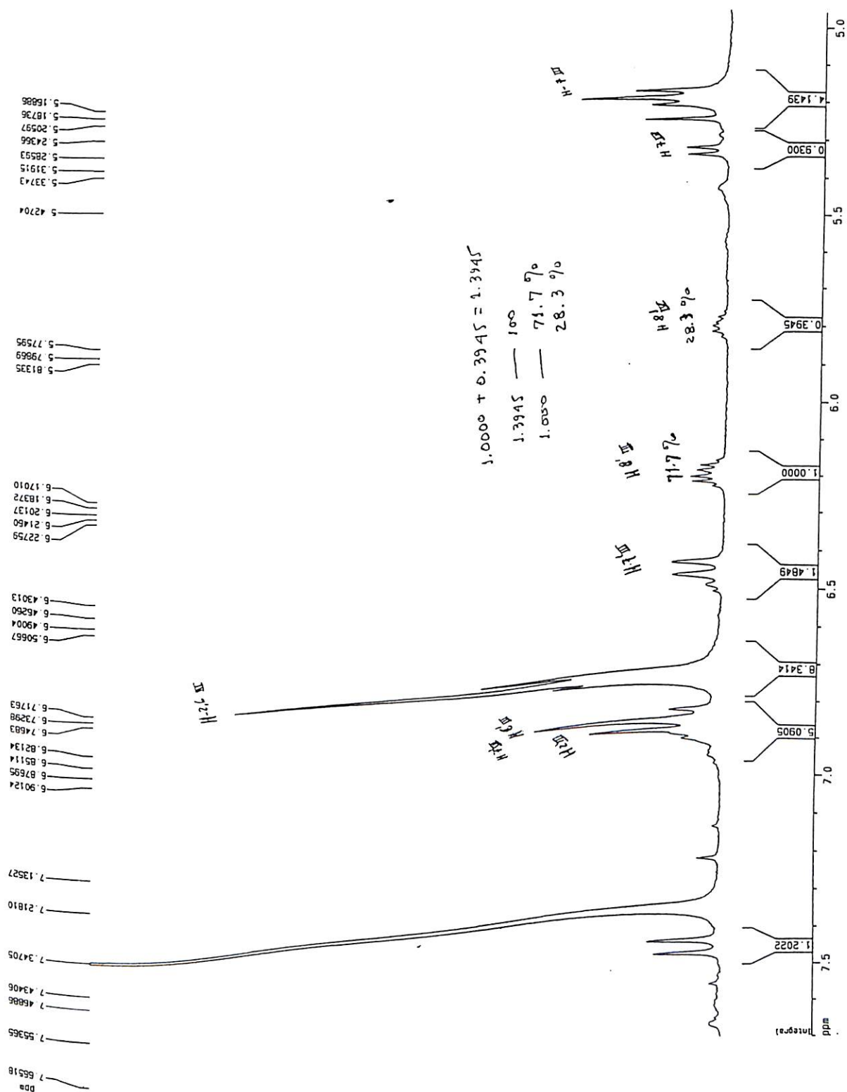
Figura 15: Espectro de RMN de ^1\text{H} , região 5,0-7,5 ppm das neolignanas III e IV (500 MHz, \text{CDCl}_3 )
