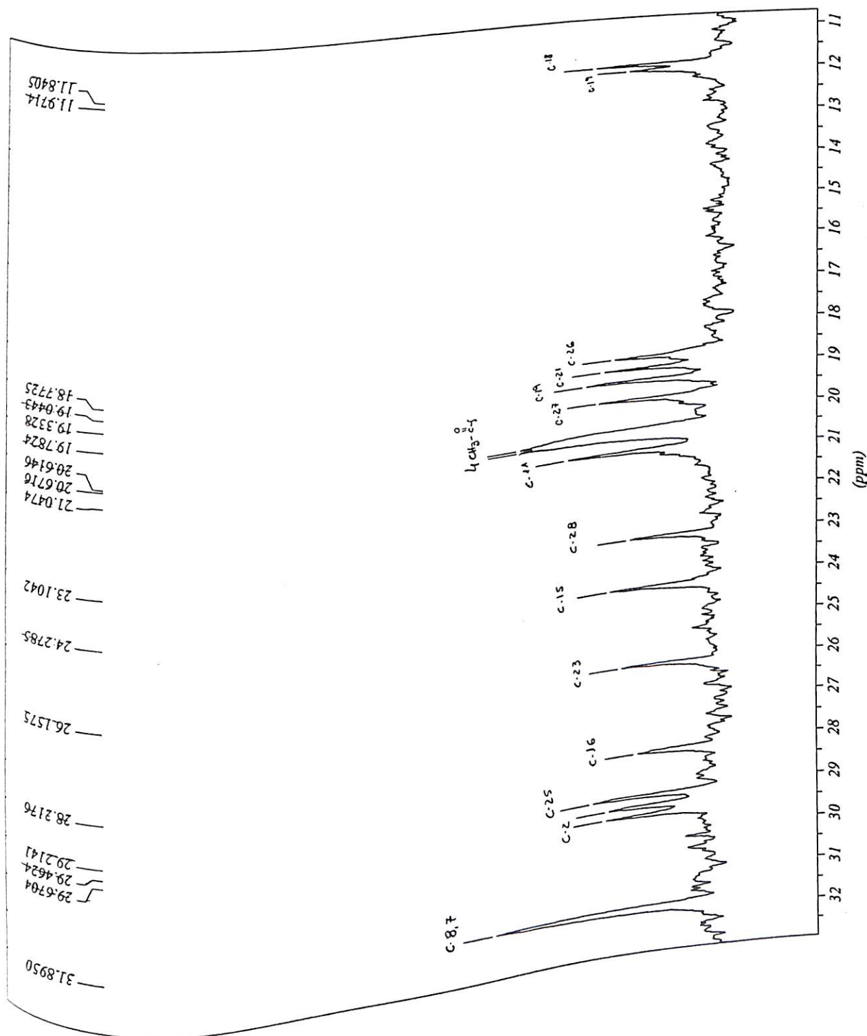
Figura 51 : Espectro de RMN de ^{13}\text{C} , região 11,0-33,0 ppm do esteroide VI (100 MHz, \text{CDCl}_3 )
