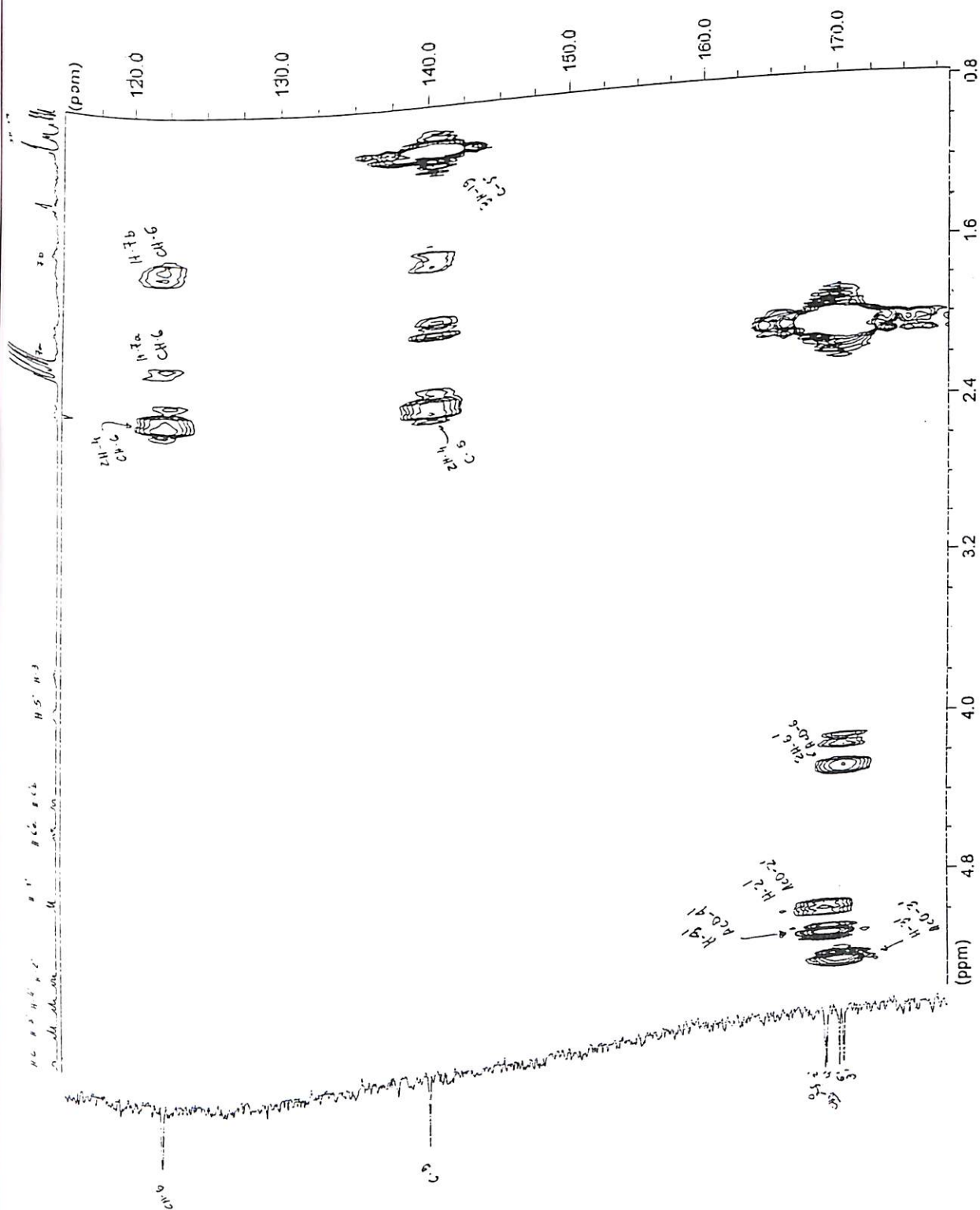
Figura 57 : Espectro de ^1\text{H} \times ^{13}\text{C} HMBC, região 0,8-5,2 x 110,0-185,0 ppm do esteroide VI (100 MHz, \text{CDCl}_3 )
