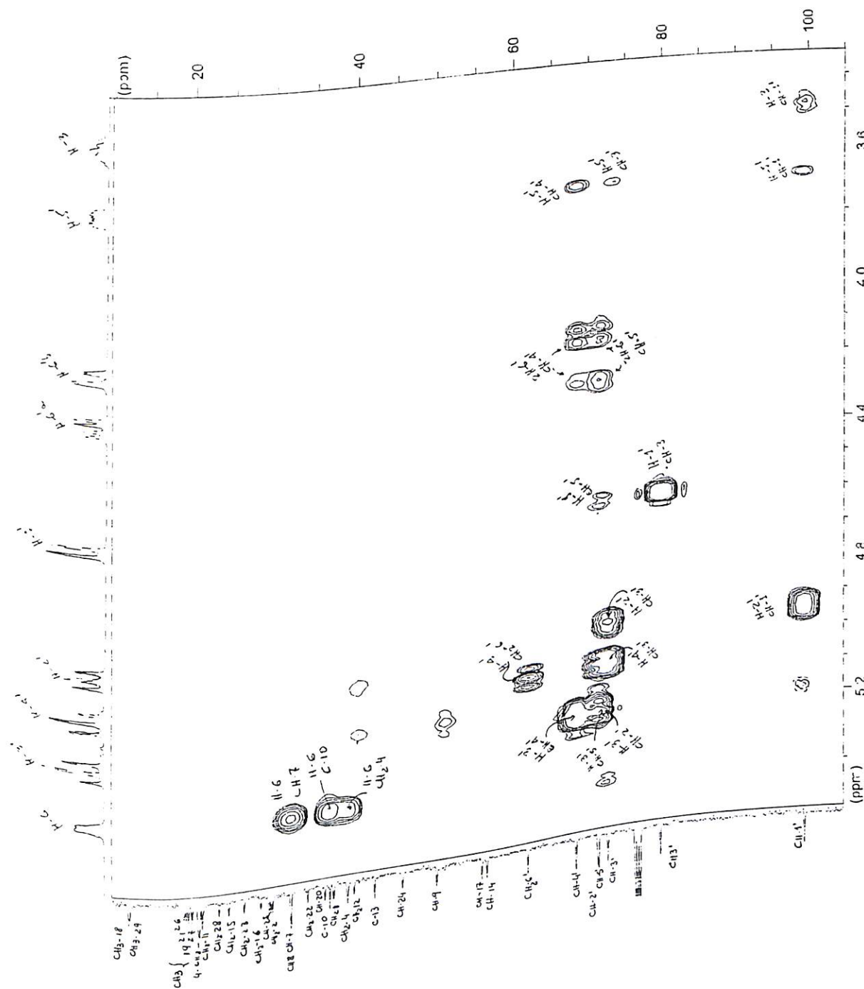
Figura 56 : Espectro de ^1\text{H} \times ^{13}\text{C} HMBC, região 3,4-5,6 x 10,0-105,0 ppm do esteróide VI (100 MHz, \text{CDCl}_3 )
