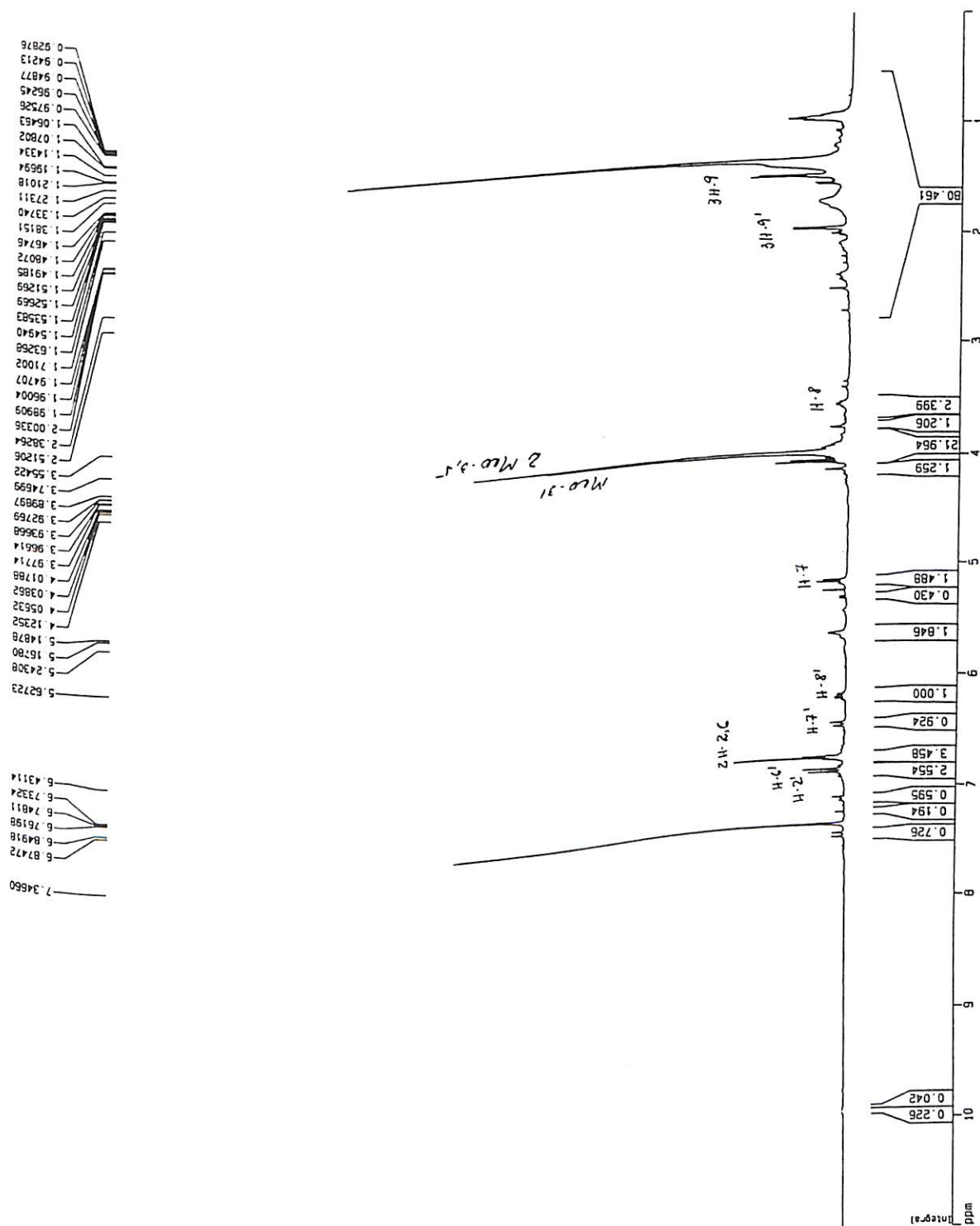
Figura 29 : Espectro de RMN de ^1\text{H} da neolignana V (500 MHz, \text{CDCl}_3 )
