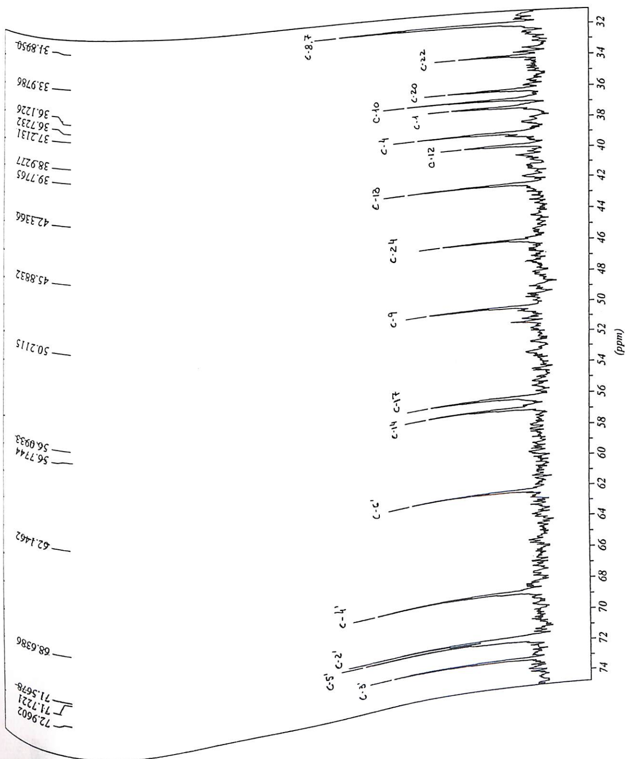
Figura 52 : Espectro de RMN de ^{13}\text{C} , região 31,0-74,5 ppm do esteroide VI (100 MHz, \text{CDCl}_3 )
