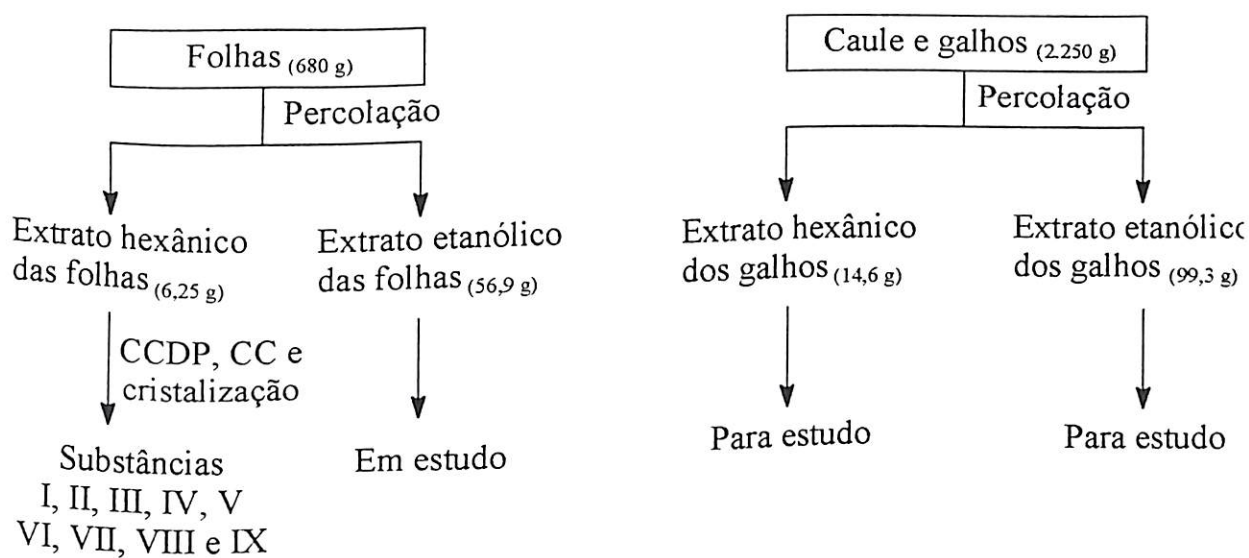
Esquema 1 : Metodologia utilizada para obtenção dos extratos e dos constituintes químicos das folhas de N. membranacea (Spreng.) Hassler.
