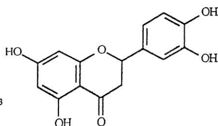
15a : \Delta^{2,3} 15b : 2,3 diidro
