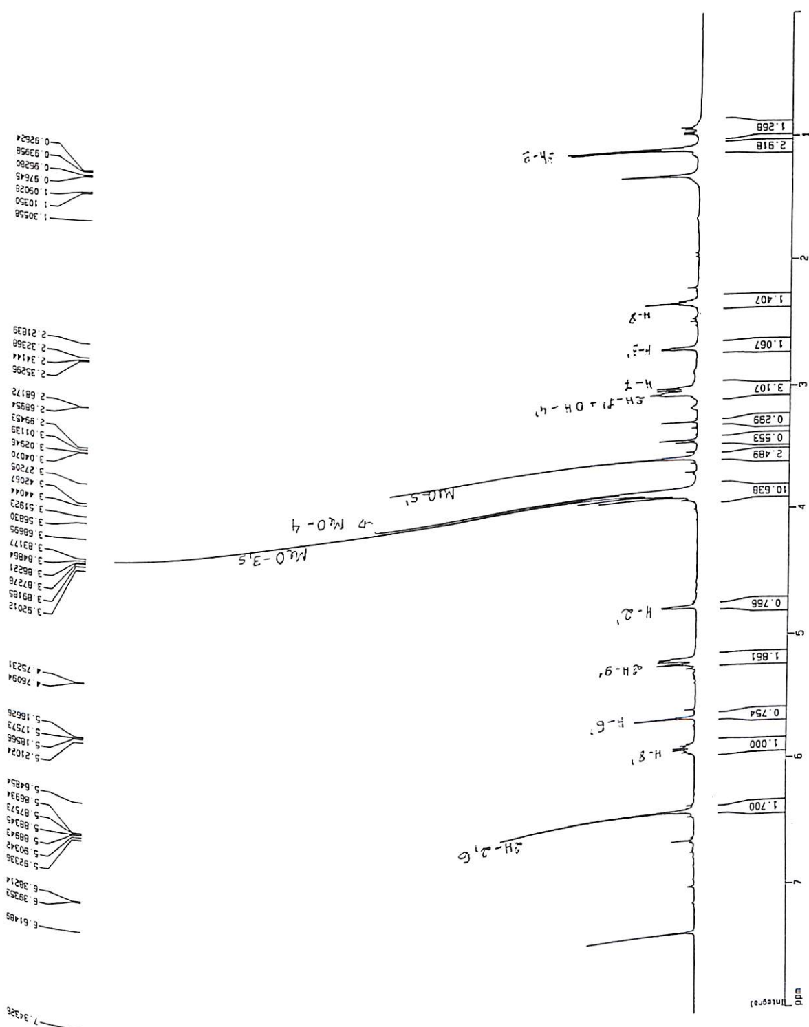
Figura 59 : Espectro de RMN ^1\text{H} da neolignana VII (500 MHz, \text{CDCl}_3 )
