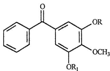
9 : R = R 1 = H - Cotoína 9a : R = H; R 1 = CH 3 9b : R = R 1 = C 2 H 5 } derivados
