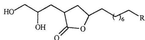
5a: R = CH 2 =CH- 5b: R = HC≡C- } Rubrenolídeo
