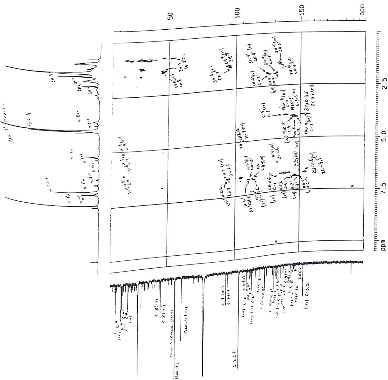
Figura 23 : Espectro de HMBC ^1\text{H} x ^{13}\text{C} - ^n\text{J}_{\text{CH}} n = 2, 3, região 0,0-10,0 x 0,0-200,0 das neolignanas III e IV (125 MHz, \text{CDCl}_3 )
