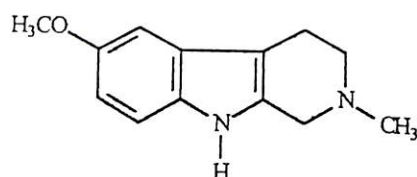
17 : 6-metoxi-N-metil-1,2,3,4-tetrahidro- \beta -carbolina
