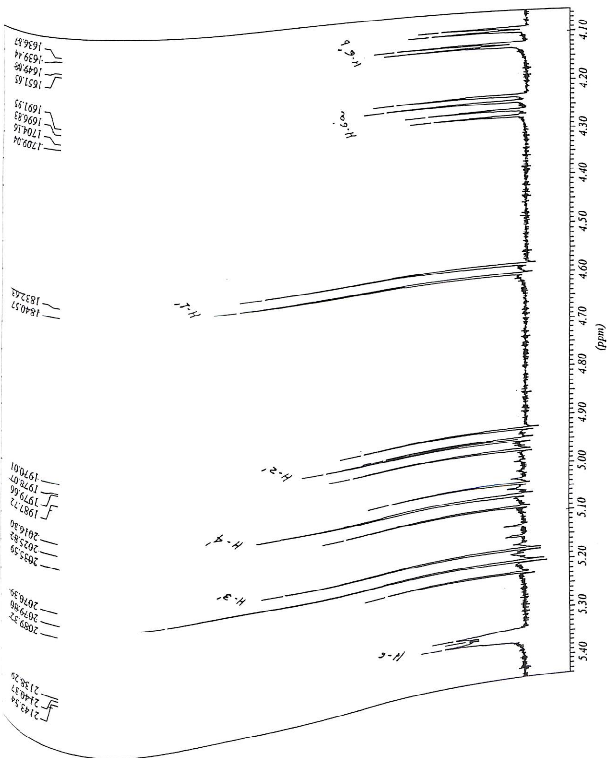
Figura 49 : Espectro de RMN de ^1\text{H} , região 4,05-5,45 ppm do esteroide VI (400 MHz, \text{CDCl}_3 )
