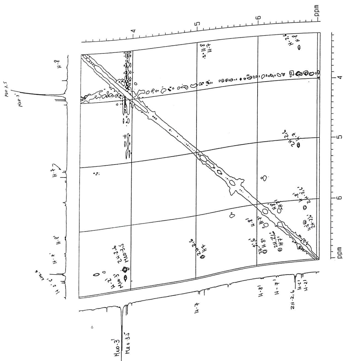
Figura 45 : Espectro de NOESY, região 3,2-7,0 x 3,2-7,0 ppm da neolignana V (500 MHz, CDCl 3 )
