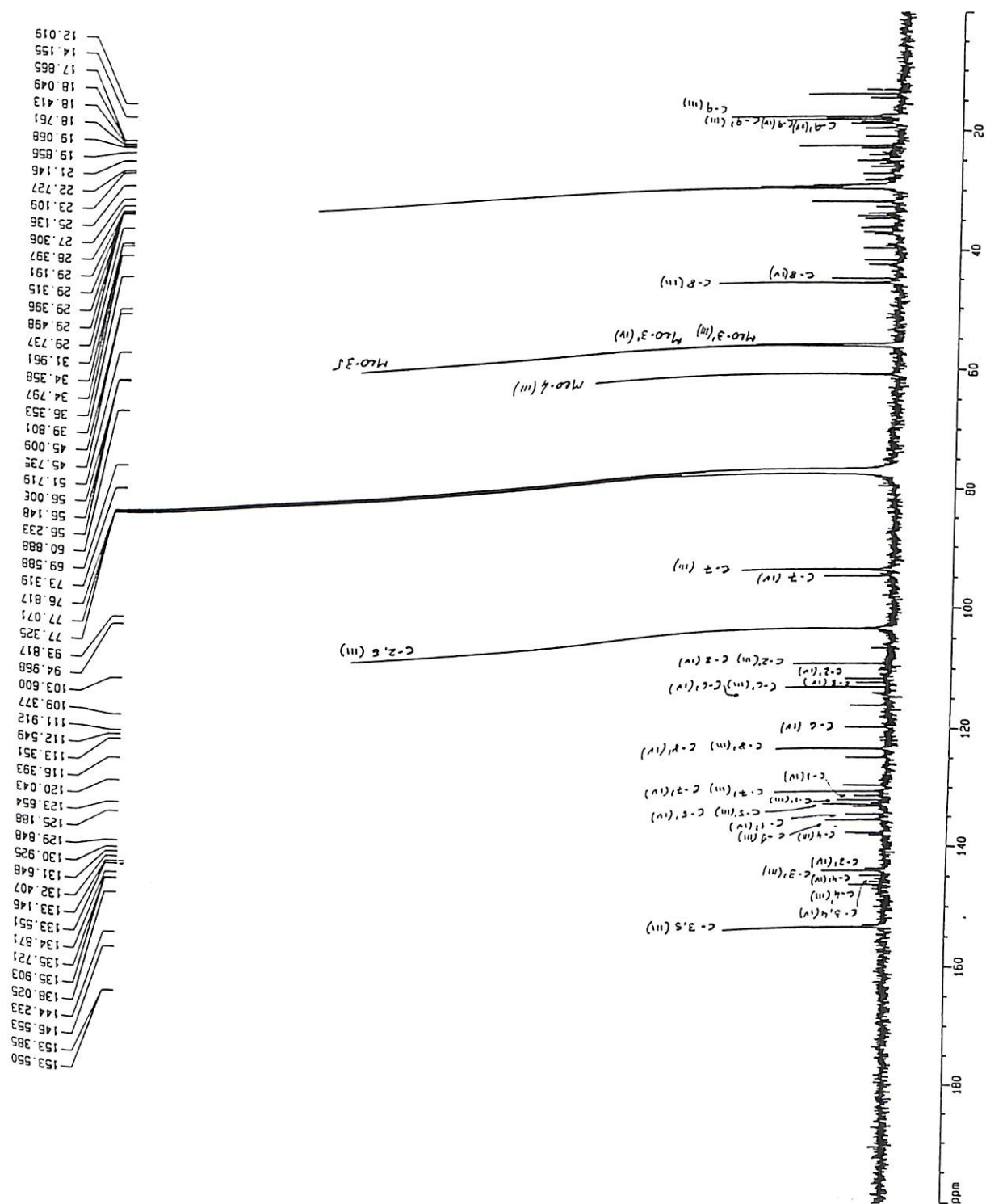
Figura 16 : Espectro de RMN de ^{13}\text{C} das neolignanas III e IV (125 MHz, \text{CDCl}_3 )
