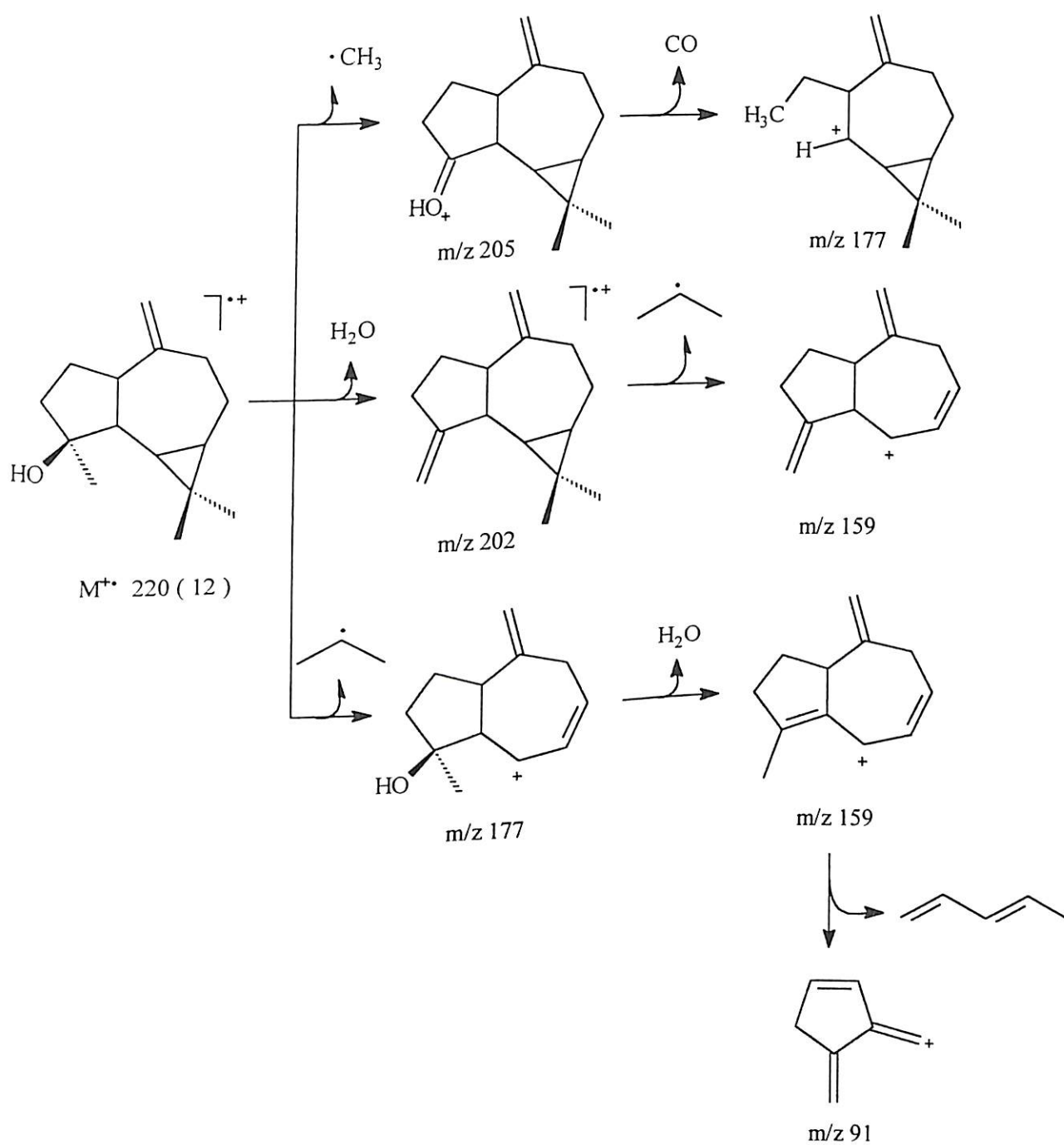
Esquema 2 : Proposta de fragmentação para o sesquiterpeno I
