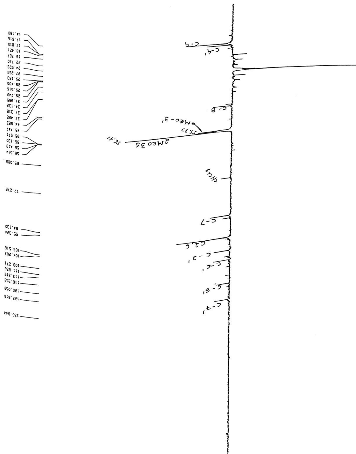
Figura 34 : Espectro de RMN de ^{13}\text{C} - DEPT 135° da neolignana V (125 MHz, \text{CDCl}_3 )
