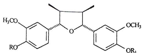
52 : R = R 1 = CH 3 - Galgravina
