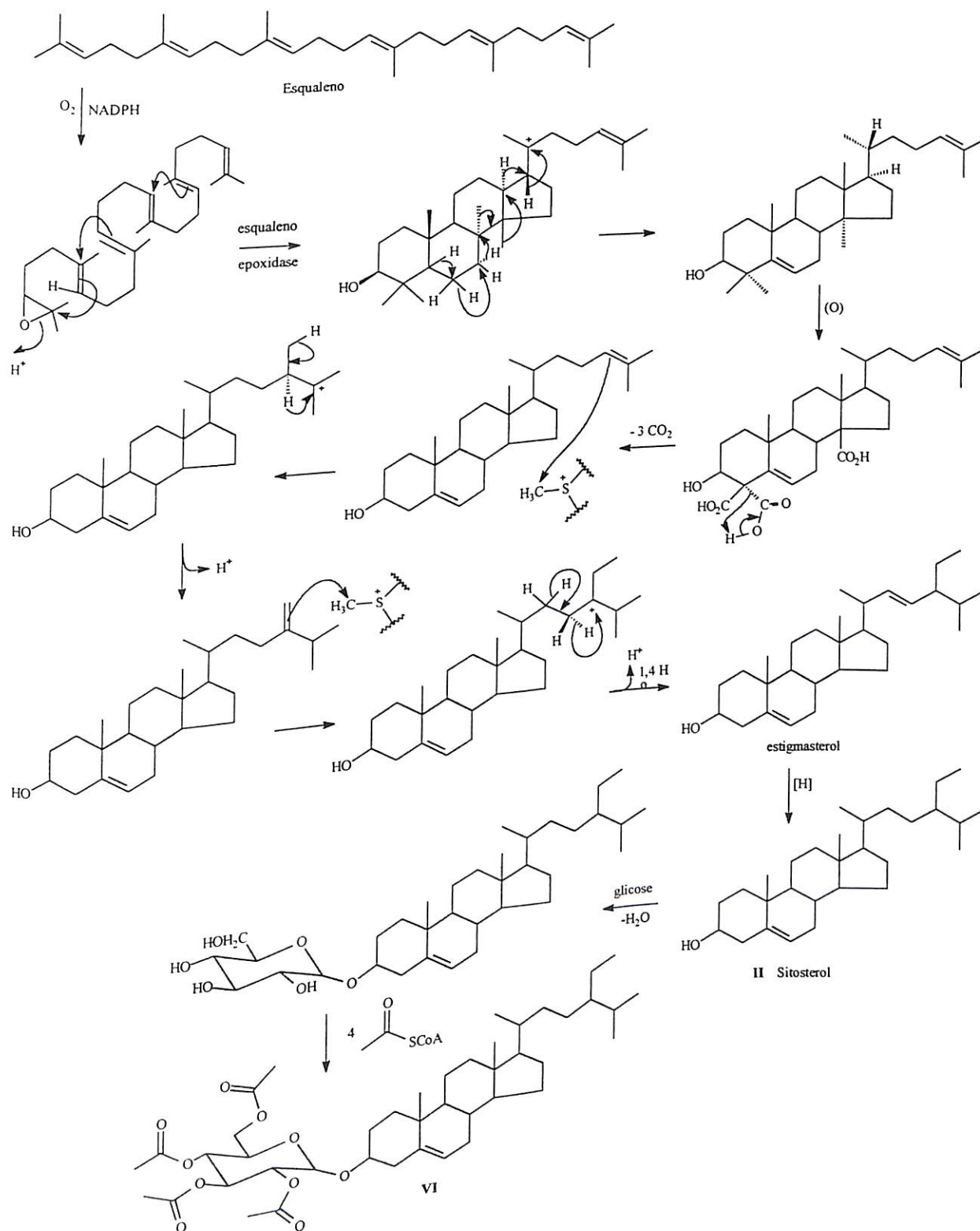
Esquema 9 : Proposta biossintética para formação das substâncias II e VI.
