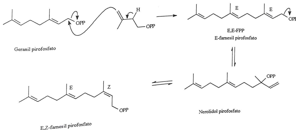
Esquema 7 : Formação das unidades farnesil e nerolidol pirofosfato.
