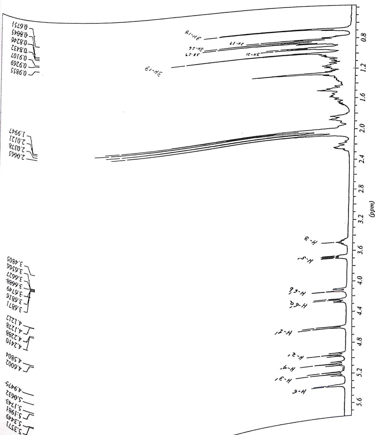
Figura 48 : Espectro de RMN de 1 H do esteroide VI (400 MHz, CDCl 3 )
