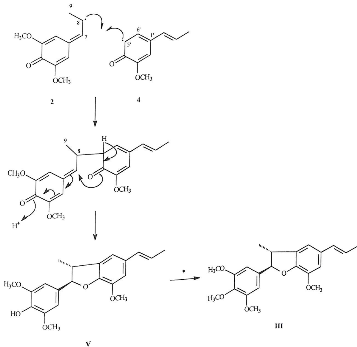
Esquema 11 : Proposta biossintética para a formação das substâncias III e V através do acoplamento oxidativo entre as unidades (2 e 4) esqueleto 8.5'
