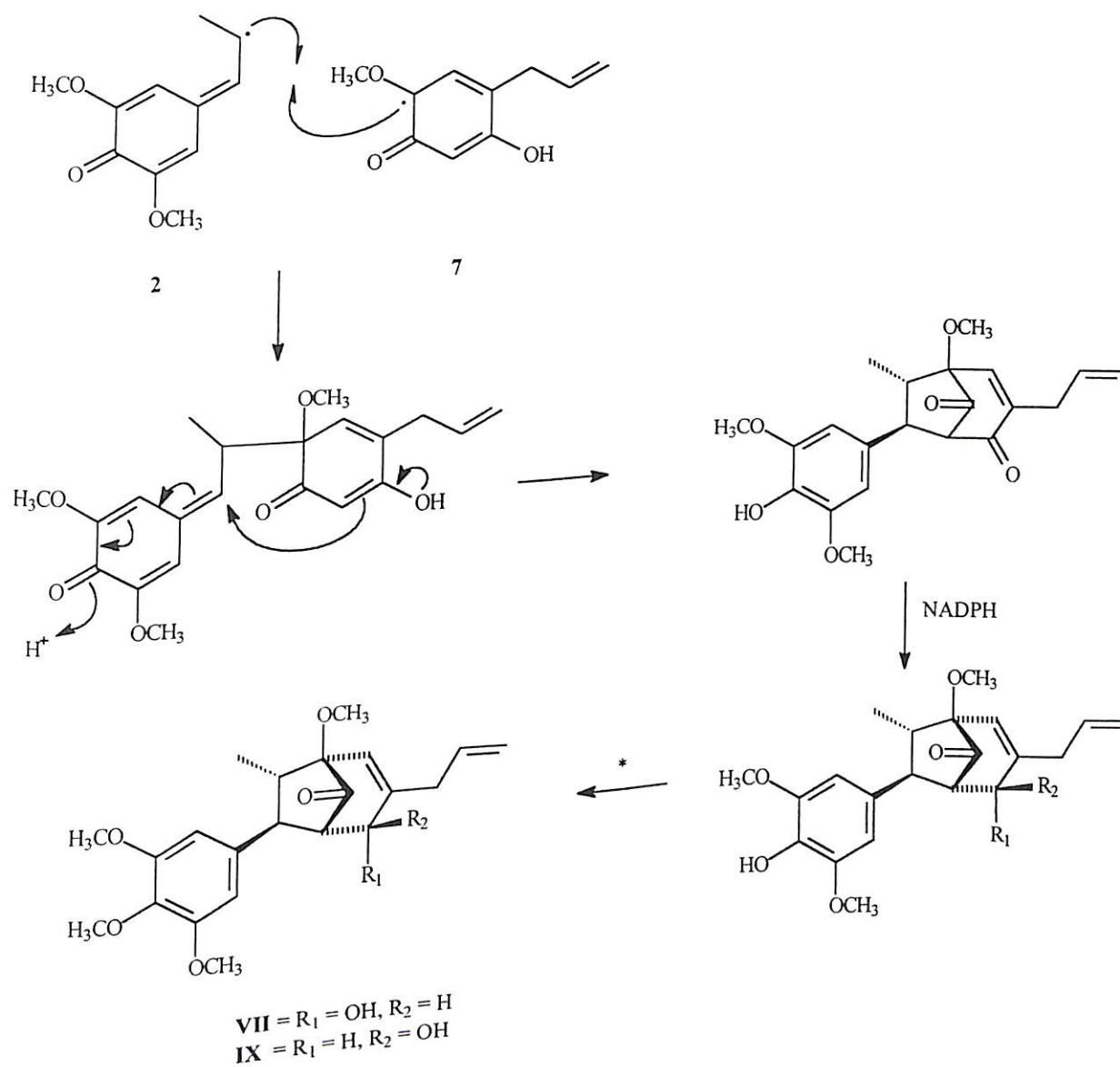
Esquema 13 : Proposta biossintética para a formação da substância VII e IX , através do acoplamento oxidativo entre as unidades (2 e 7) esqueleto 8.5'.
