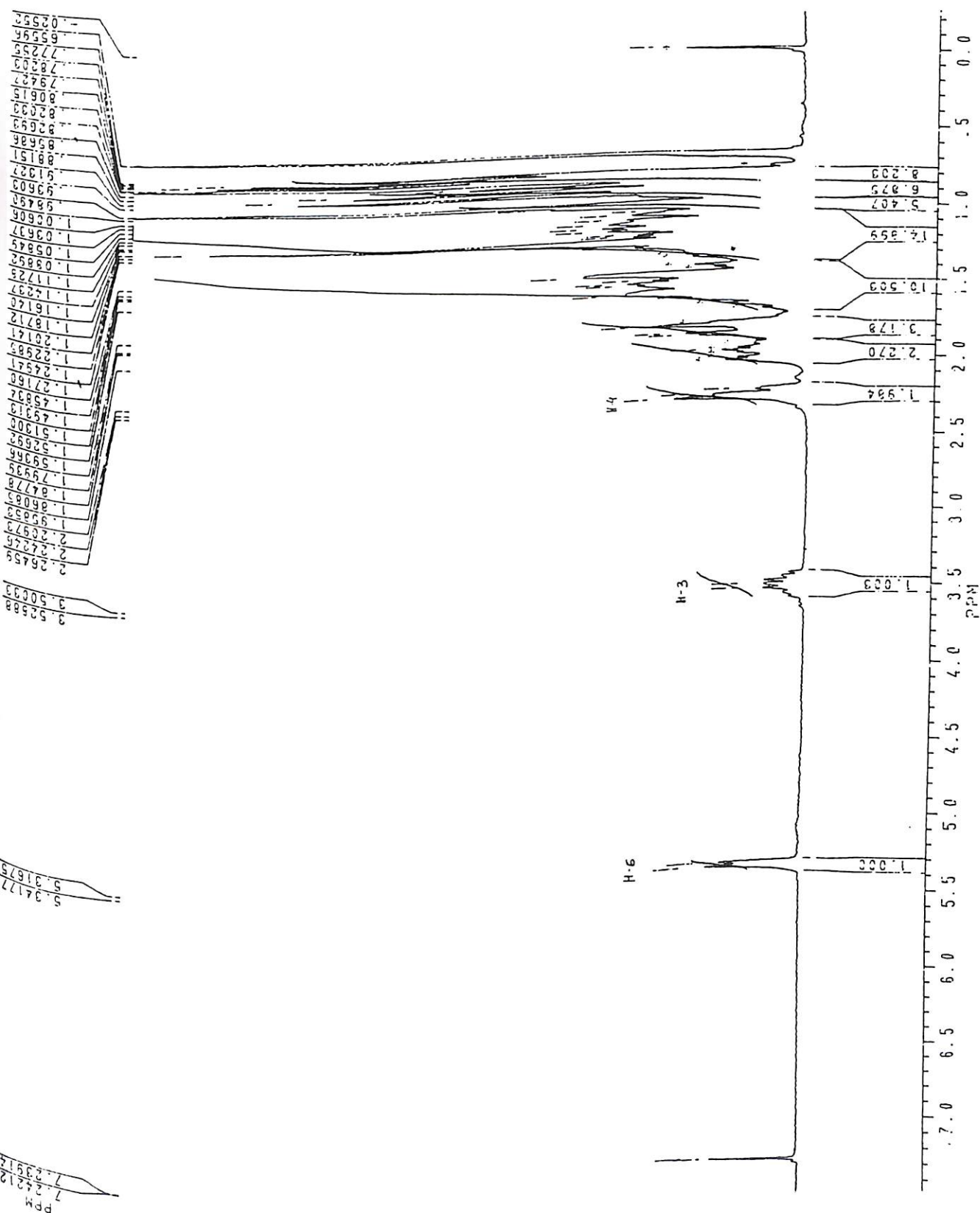
Figura 10 : Espectro de RMN de ^1\text{H} do esteroide II (200 MHz, \text{CDCl}_3 )
