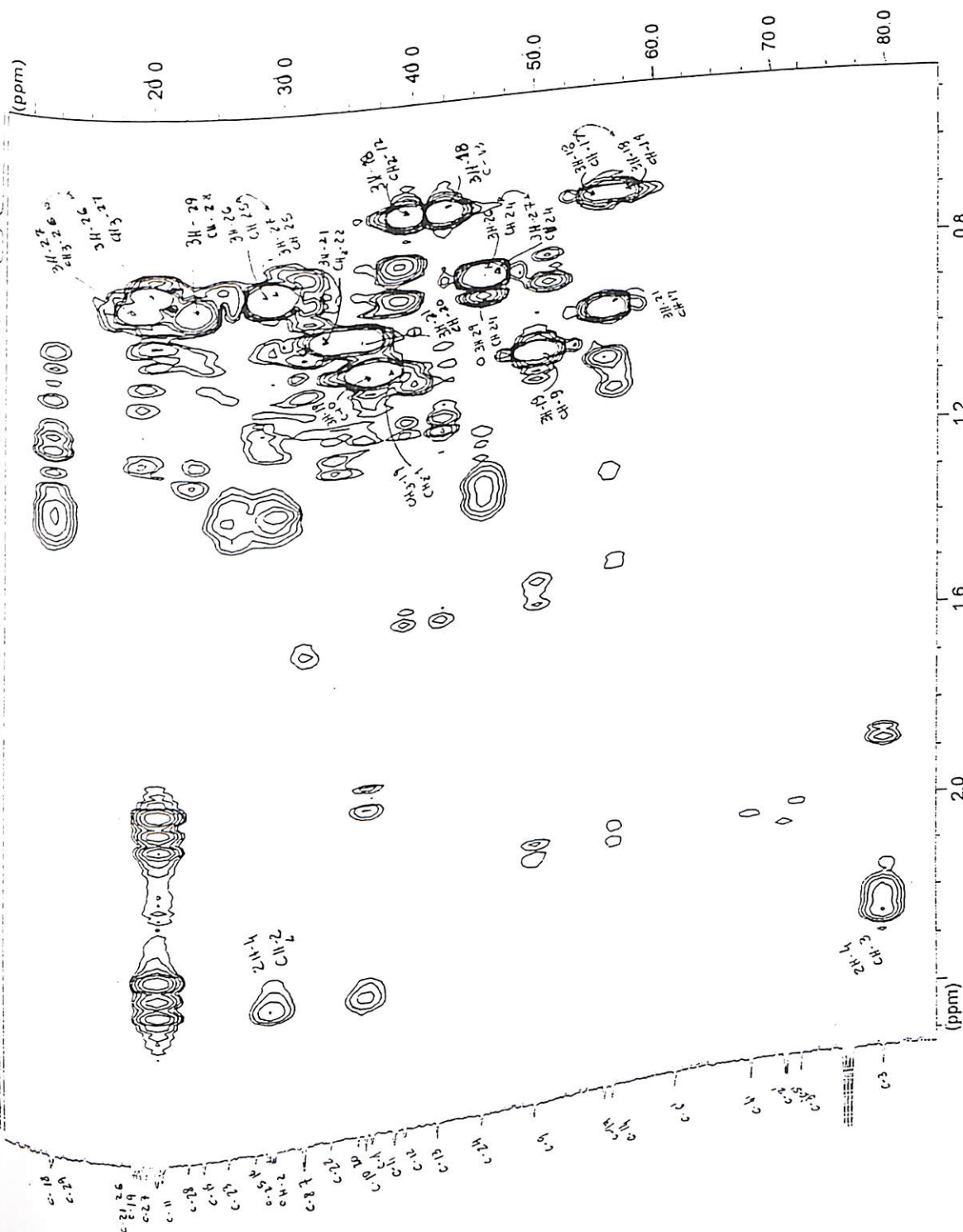
Figura 55 : Espectro de ^1\text{H} x ^{13}\text{C} HMBC, região 0,3-2,5 x 10,0-85,0 ppm do esteroide VI (100 MHz, \text{CDCl}_3 )
