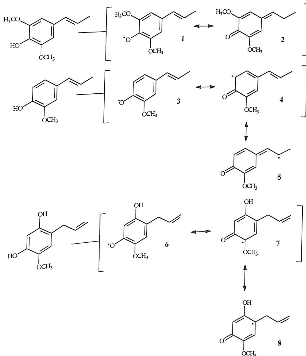
Esquema 10 : Formação de radicais de alil (6, 7 e 8) propenil fenol (1, 2, 3, 4 e 5) em neolignanas
