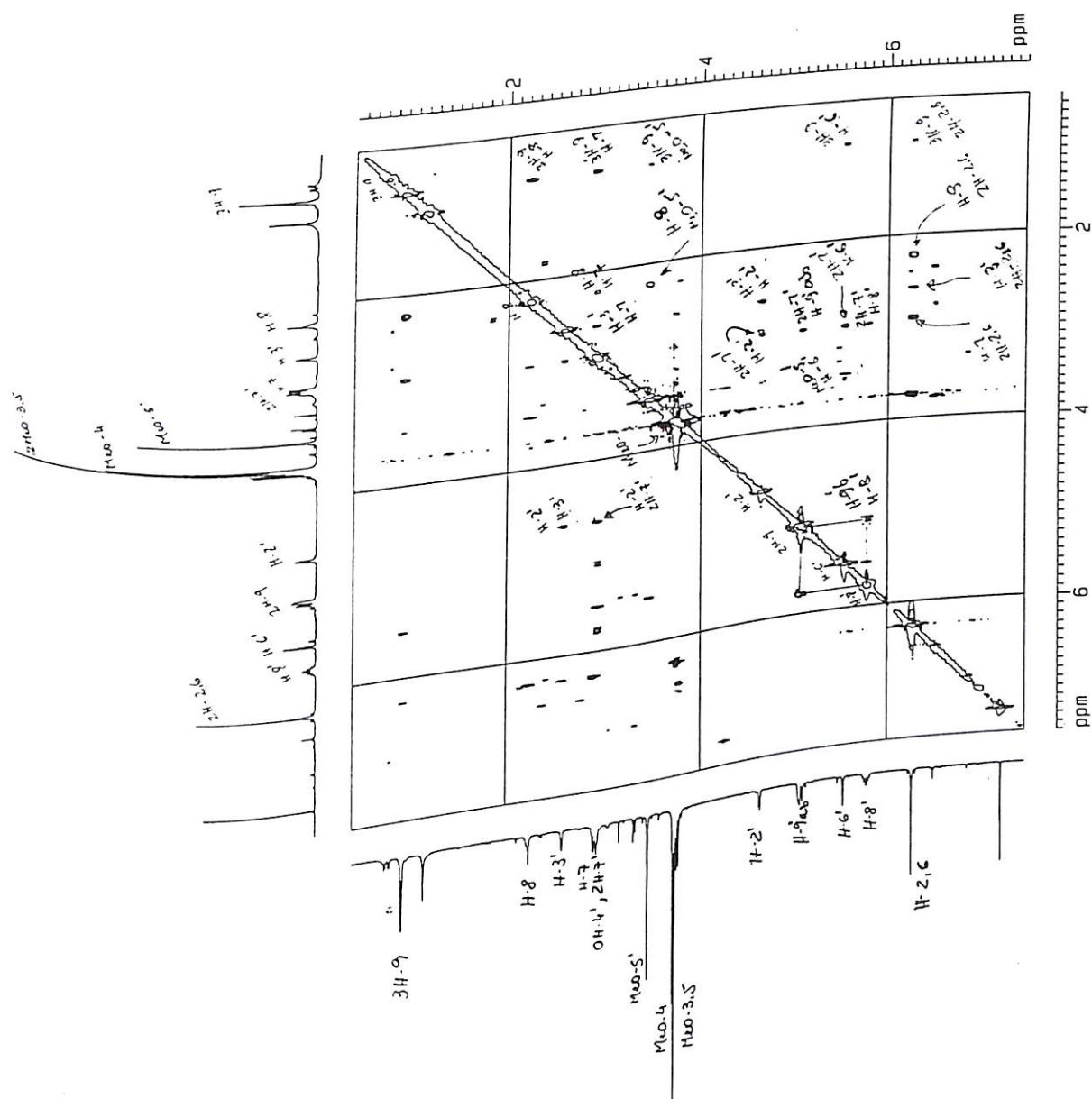
Figura 70 : Espectro de NOESY, região 1,7-7,5 x 0,0-8,0 ppm da neolignana VII (500 MHz, CDCl 3 )
