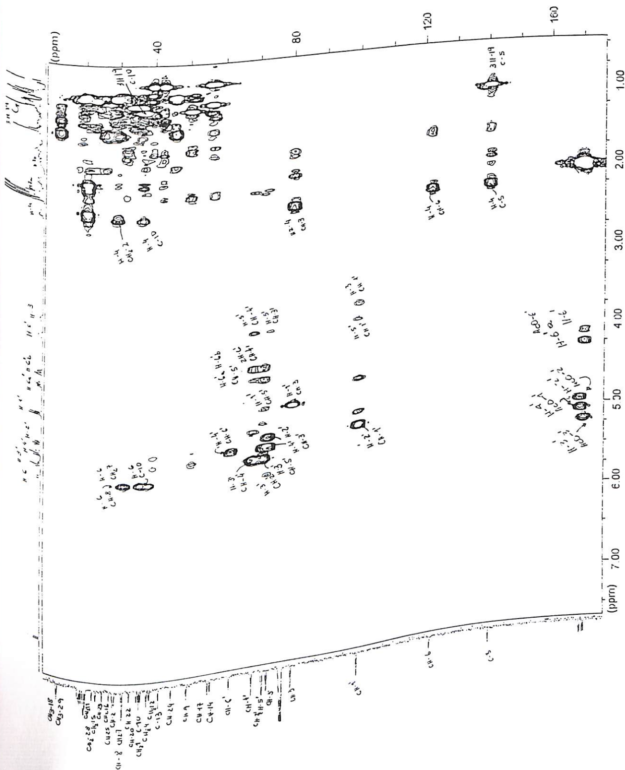
Figura 54 : Espectro de ^1\text{H} x ^{13}\text{C} HMQC, região 0,5-7,5 x 15,0-170,0 ppm do esteroide VI (100 MHz, \text{CDCl}_3 )
