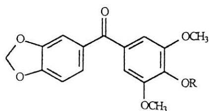
10 : R = H } 11 : R = Me } derivados
