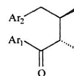
56 : Ar 1 = Pi, Ar 2 = Gu
